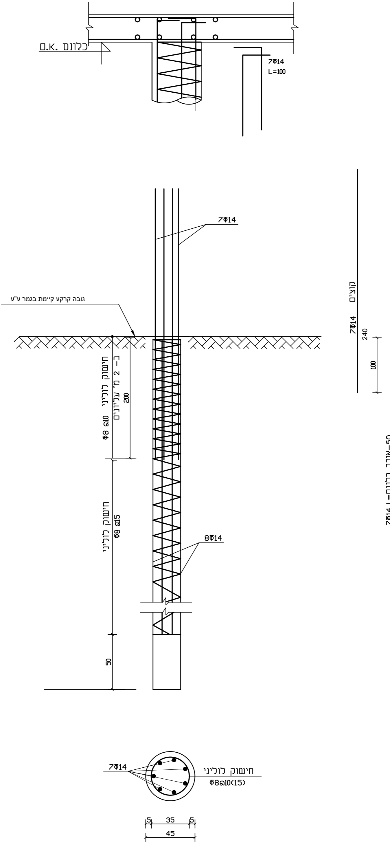
פרם לכלונס פיפוי בקוטר 45 ס"מ גודל 1:20
